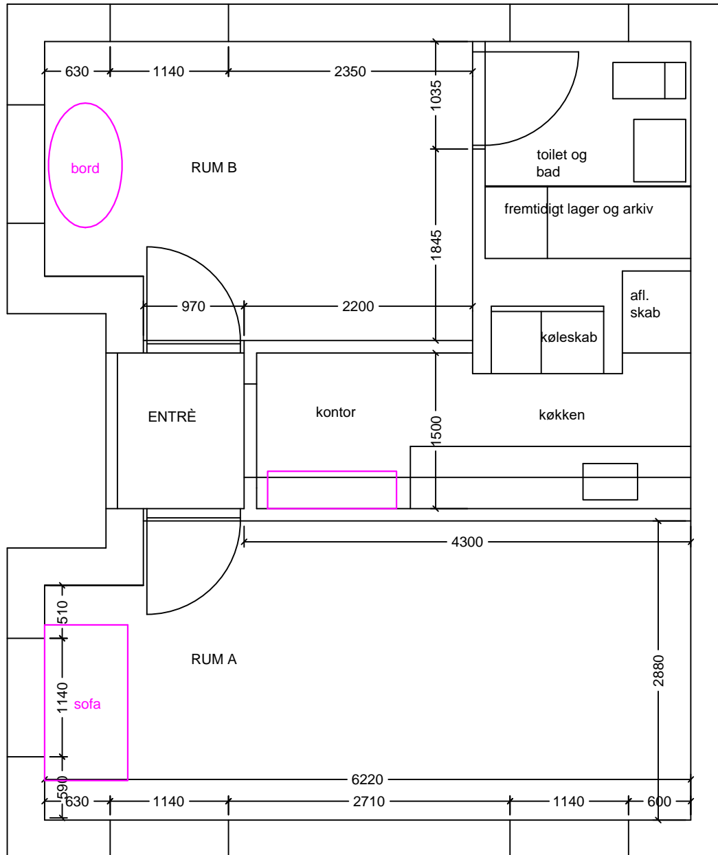
PLAN: PORTNERBOLIG . møbleret. Mål 1:50, Lofthøjde overalt 243 cm
